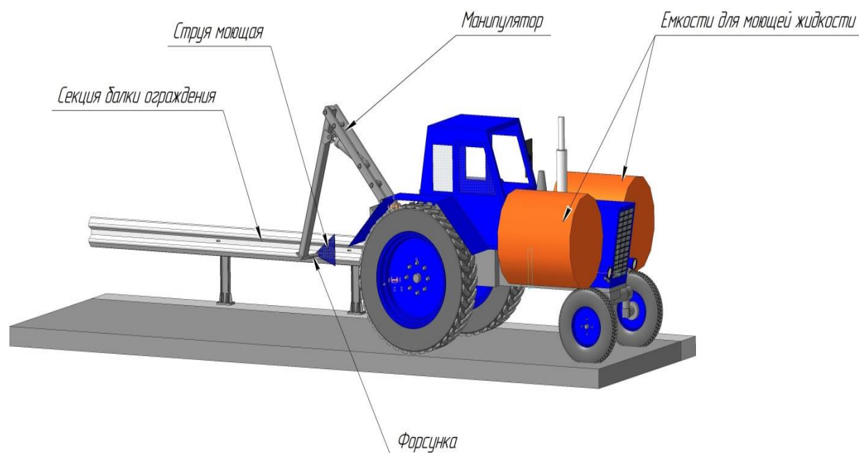
Рисунок 4 – Устройство для бесконтактной мойки дорожных ограждений
