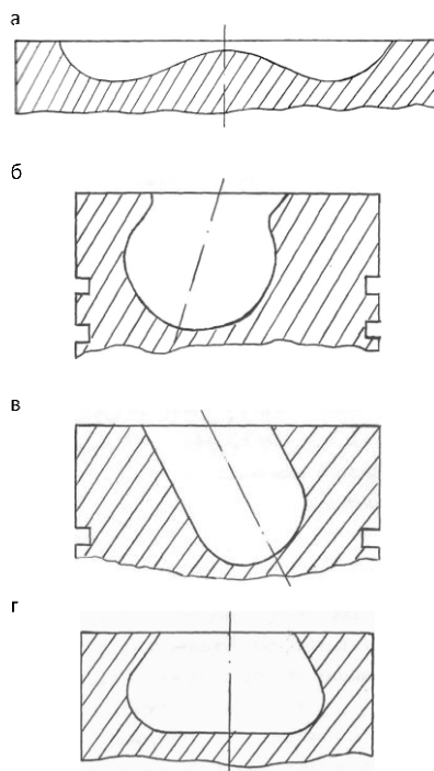
Рисунок 1 - Типы камер сгорания: а – КС типа «Гесельман»; б – КС типа «МАН»; в – КС типа «Пишингер2»; г – КС типа «ЦНИДИ»
