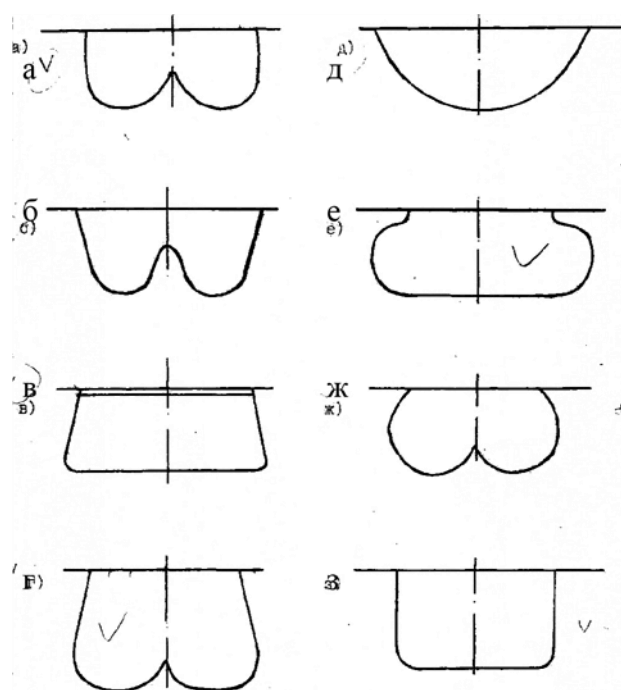
Рисунок 2 - Формы открытых камер сгорания: а – КС типа «Лейланд»; б – КС типа «Скания»; в – КС типа «Мерседес Бенц»; г – КС типа «Ивеко»; д – КС типа «Альбион»; е – КС типа «Перкинс»; ж – КС типа «Зауэр»; з – КС типа «КамАЗ»
