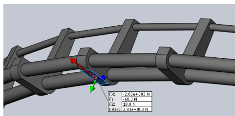
Рисунок 3. Реакция опоры места крепления каната к садку
