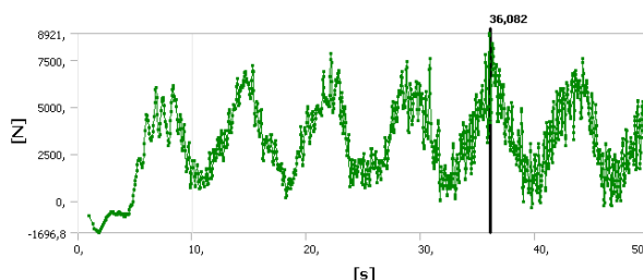
Рисунок 5. График изменения осевого усилия наиболее нагруженного каната
