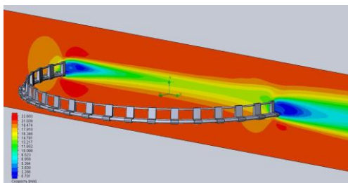
Рисунок 2. Распределение скоростей потока воздуха в диаметральной плоскости садка
